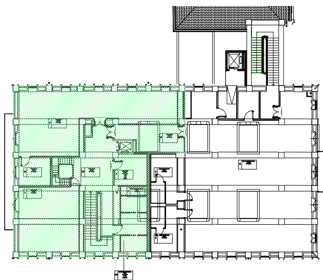
Piano secondo
